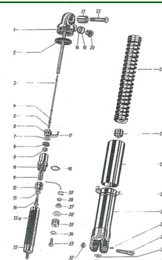
250 SG/S (1. Ausf.)
