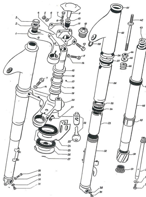
Puch 125/175 SV/S
