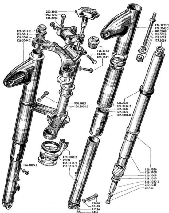
Puch 125/150 TL
