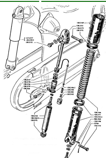
125/150 TL
