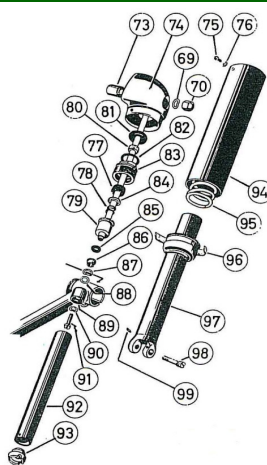
125/150 SR/A vorne
