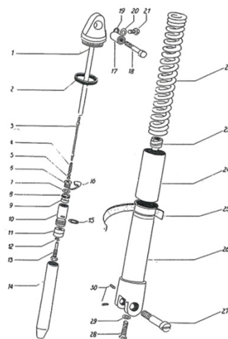
125/175 SV/S (1. Ausf.)
