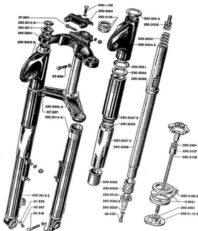
Puch 250 TF
