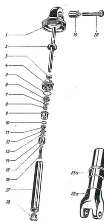
125/175 SV/S (2. Ausf.)
