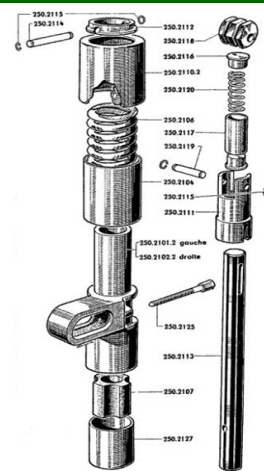
250 TF
