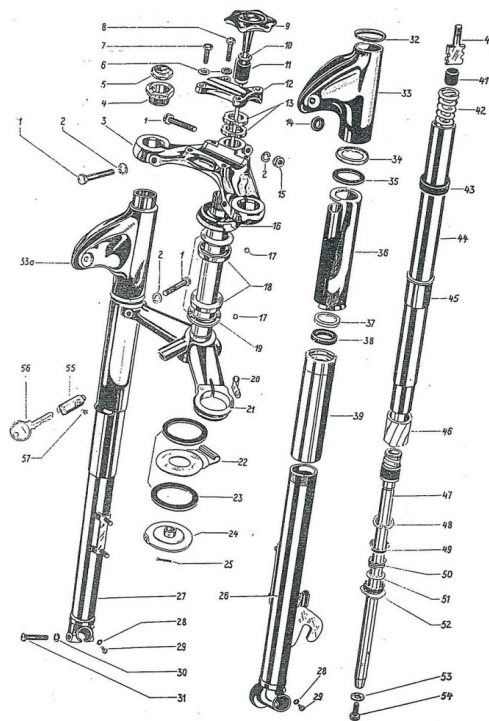
Puch 250 SG/S
